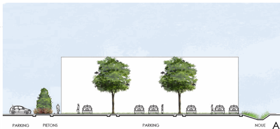
Coupe de principe des stationnements latéraux
